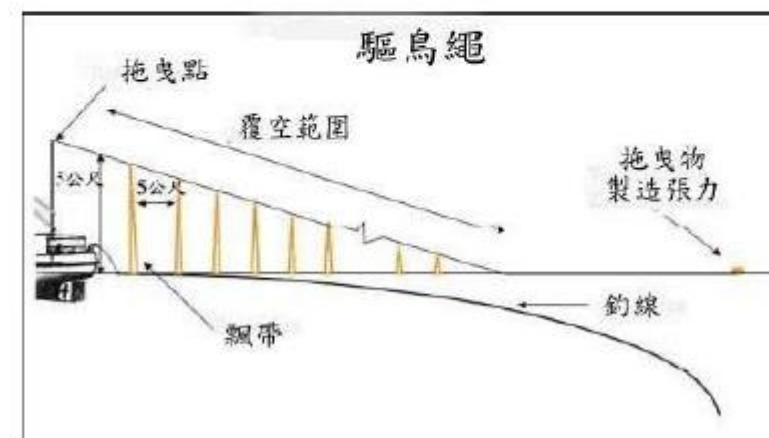
圖 驅鳥繩之概要圖示
